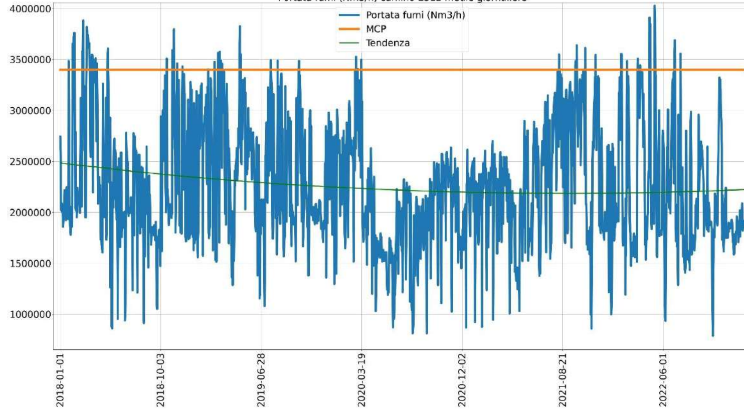
Portata fumi (Nm3/h) camino E312 medie giornaliere
