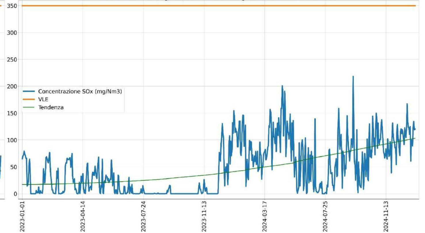
Concentrazione SOx (mg/Nm3) camino E312 medie giornaliere anno 2023 e anno 2024
