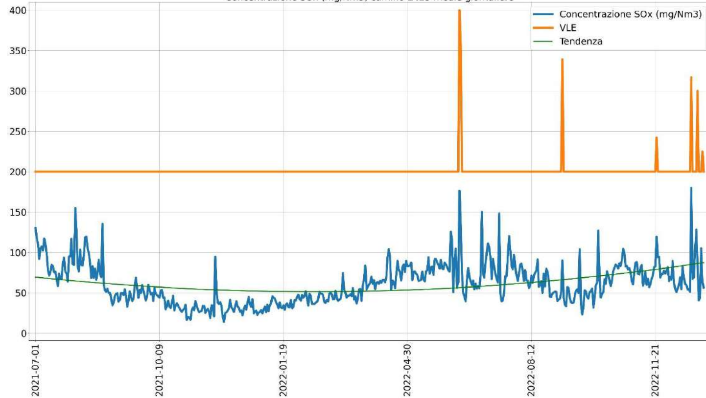
Concentrazione SOx (mg/Nm3) cammino E425 medie giornaliere
