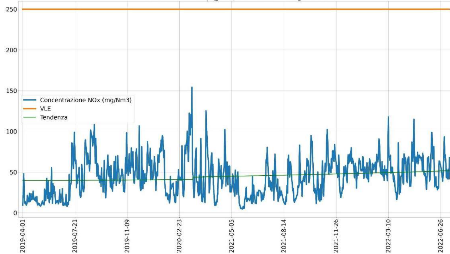
Concentrazione NOx (mg/Nm3) cammino E135 medie giornaliere
