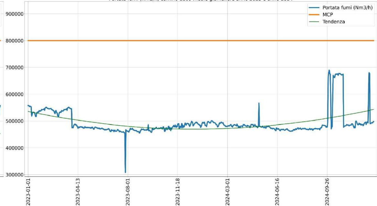
Portata fumi (Nm3/h) camino E109 medie giornaliere anno 2023 e anno 2024
