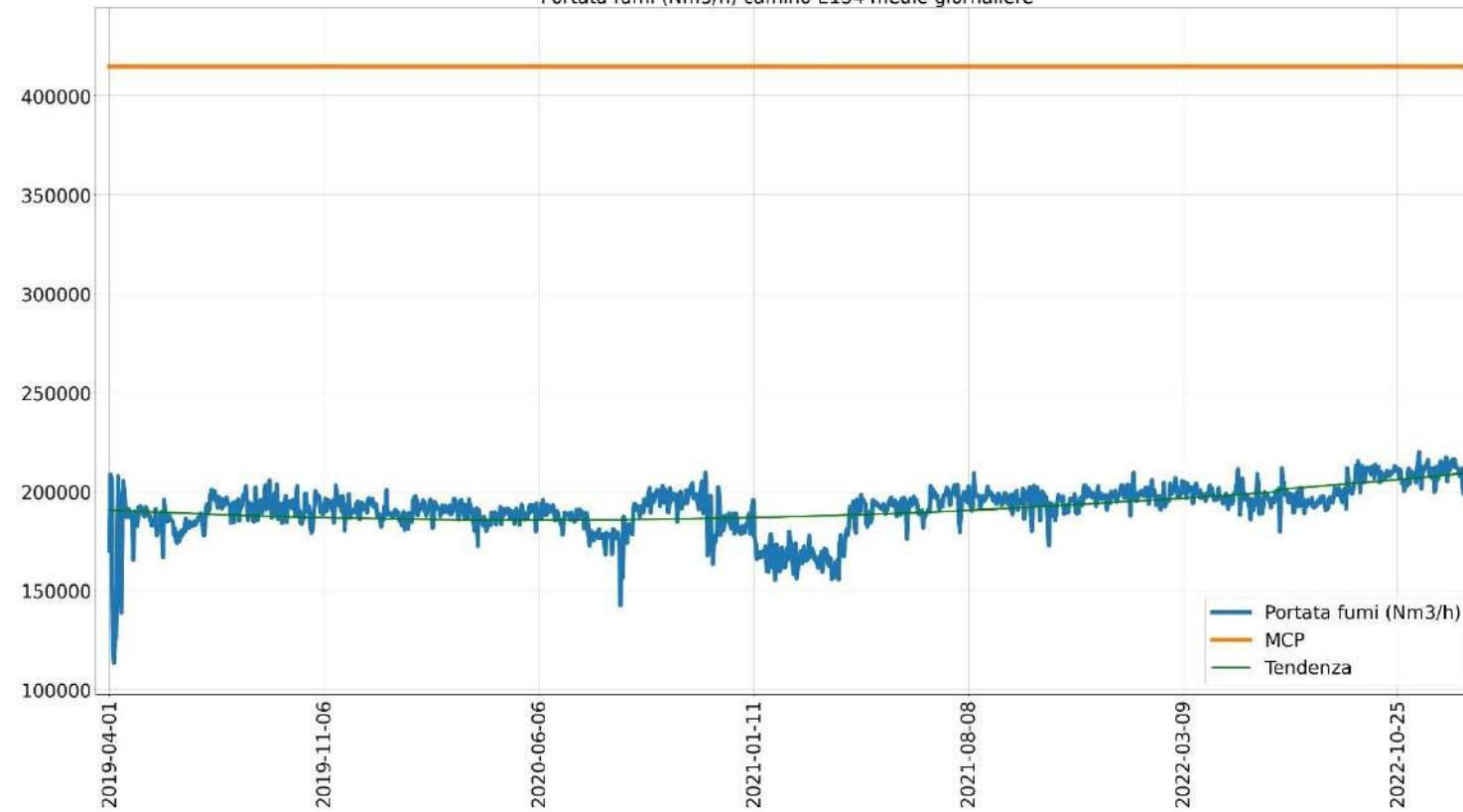
Portata fumi (Nm 3 /h) camino E134 medie giornaliere
