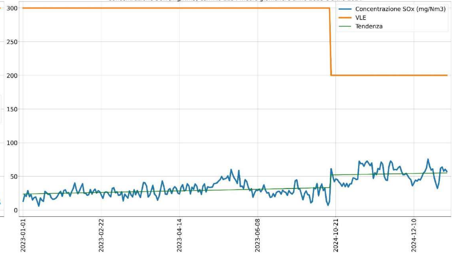
Concentrazione SOx (mg/Nm3) camino E134 medie giornaliere anno 2023 e anno 2024
