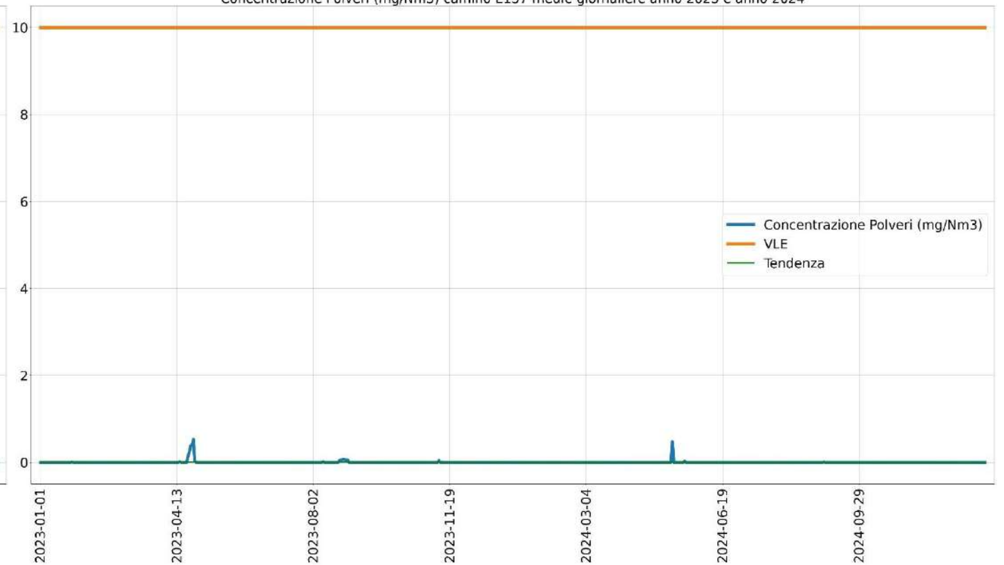
Concentrazione Polveri (mg/Nm 3 ) camino E137 medie giornaliere anno 2023 e anno 2024
