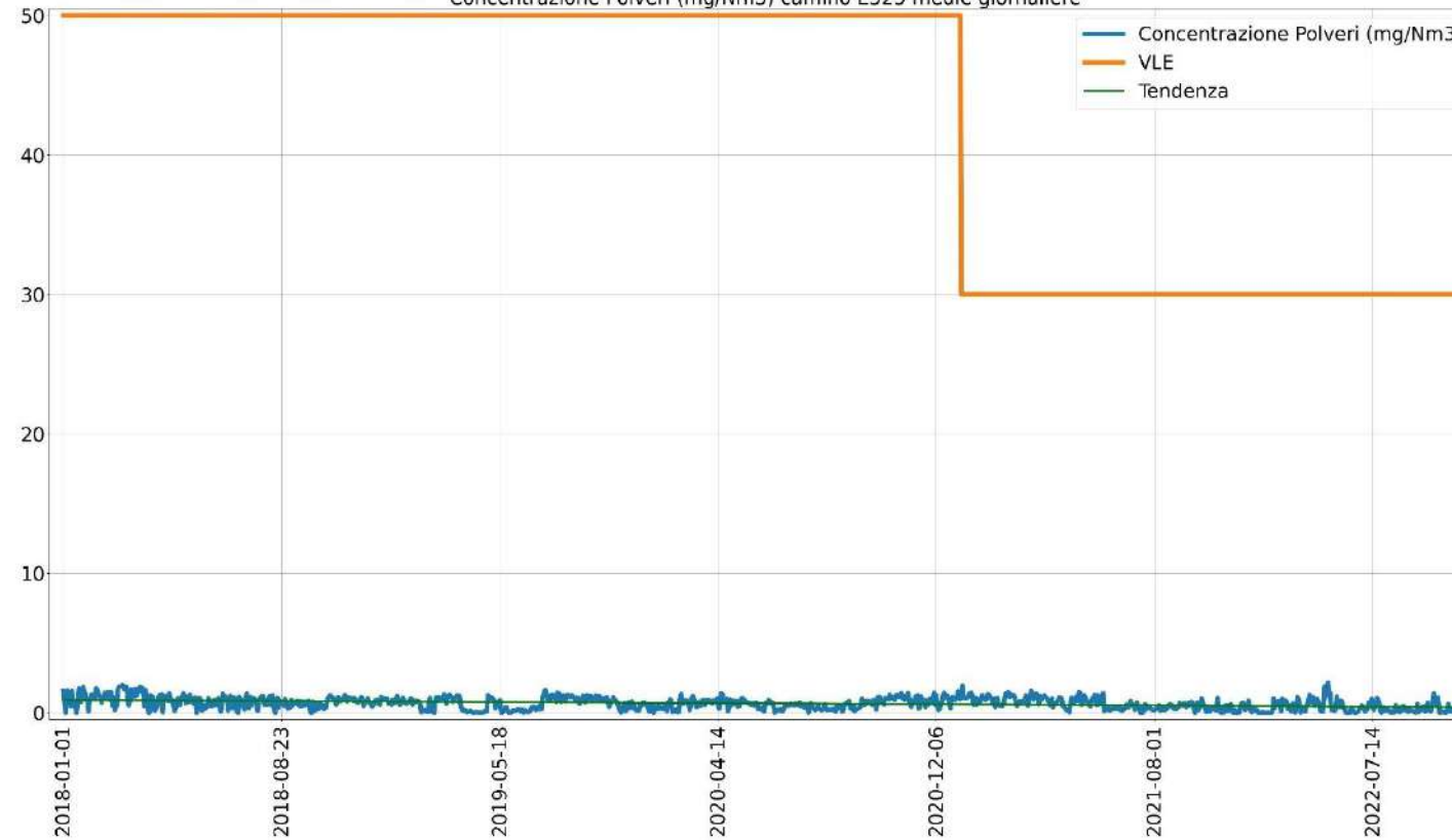
Concentrazione Polveri (mg/Nm 3 ) camino E325 medie giornaliere
