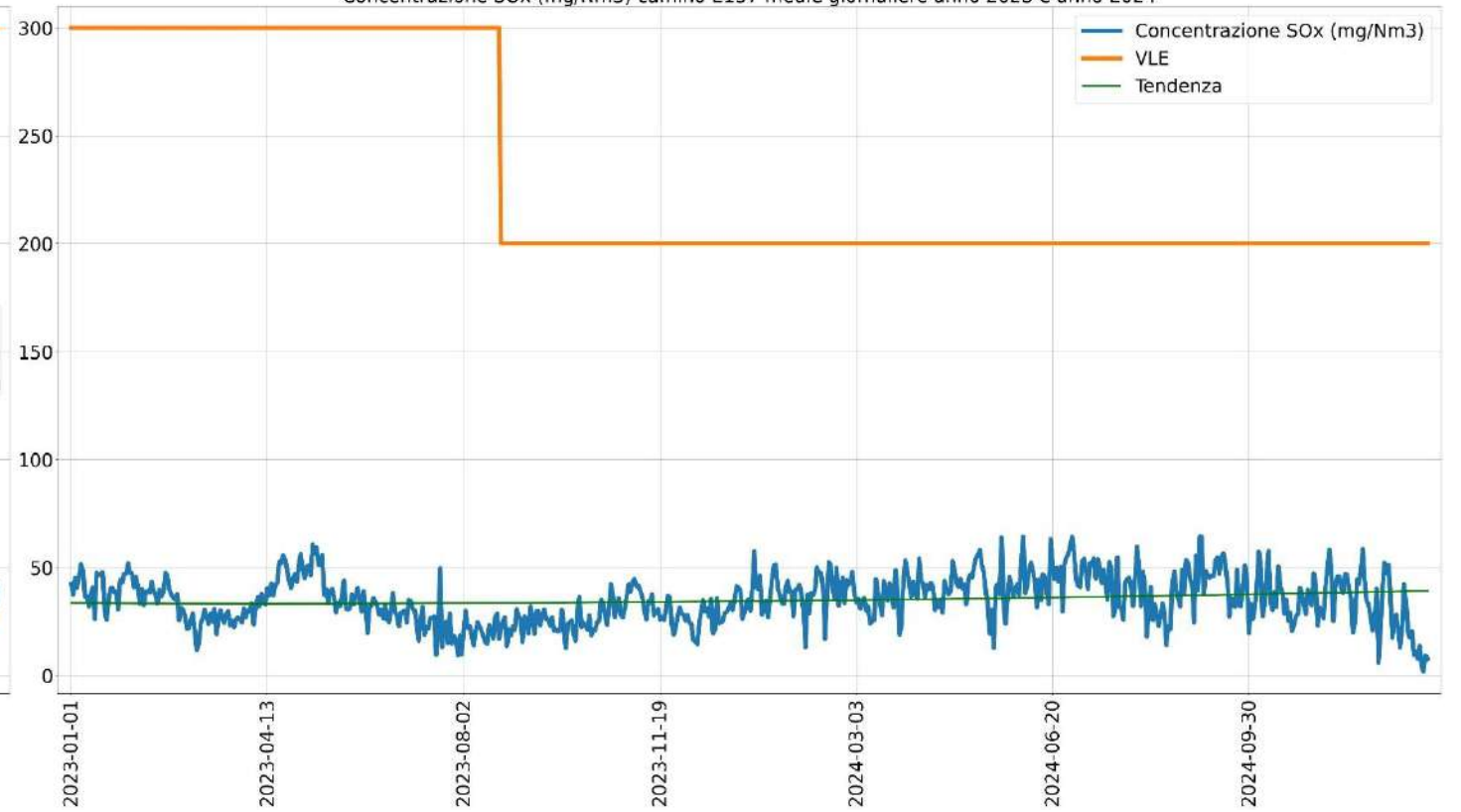
Concentrazione SOx (mg/Nm3) camino E137 medie giornaliere anno 2023 e anno 2024
