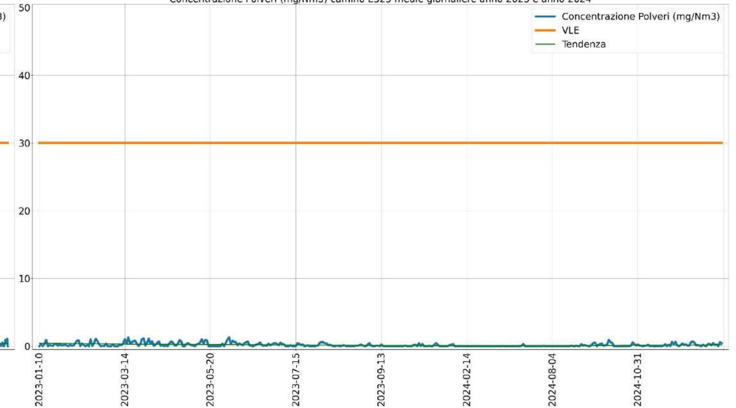
Concentrazione Polveri (mg/Nm 3 ) camino E325 medie giornaliere anno 2023 e anno 2024
