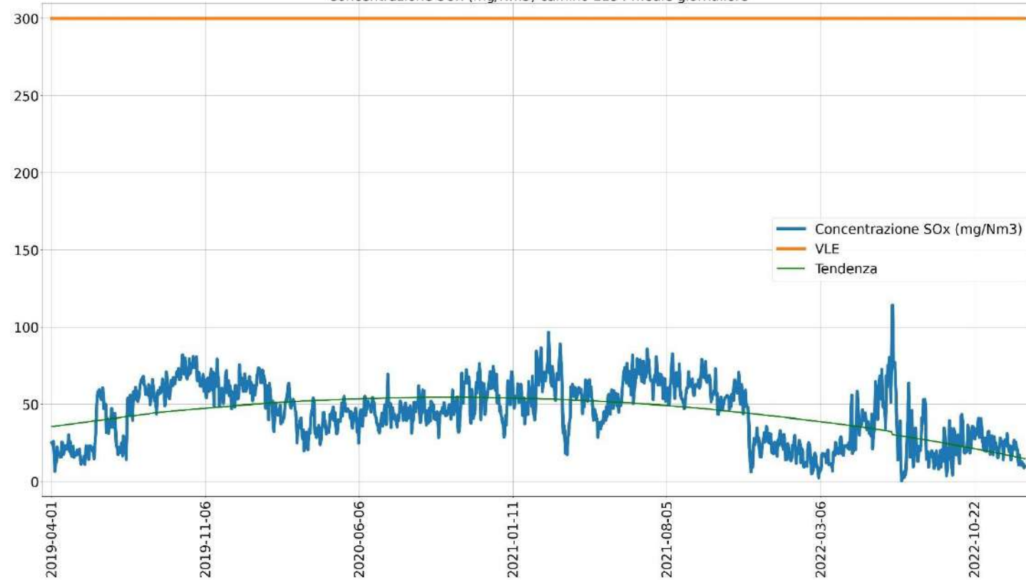
Concentrazione SOx (mg/Nm3) camino E134 medie giornaliere
