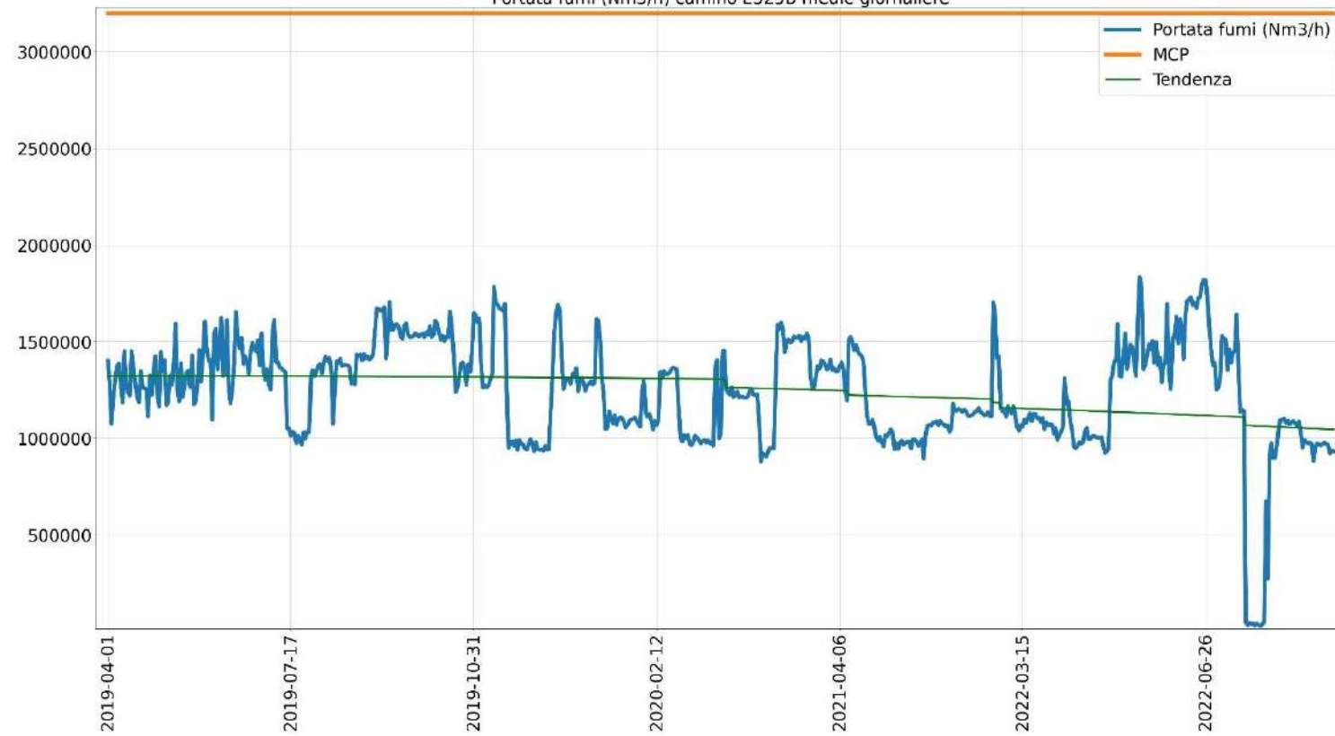
Portata fumi (Nm3/h) camino E525B medie giornaliere
