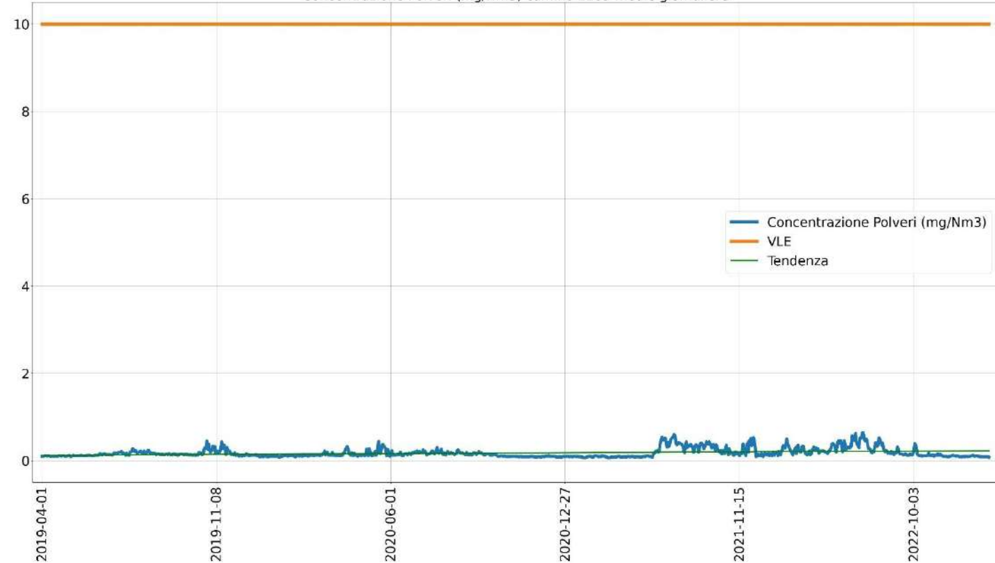
Concentrazione Polveri (mg/Nm3) camino E109 medie giornaliere
