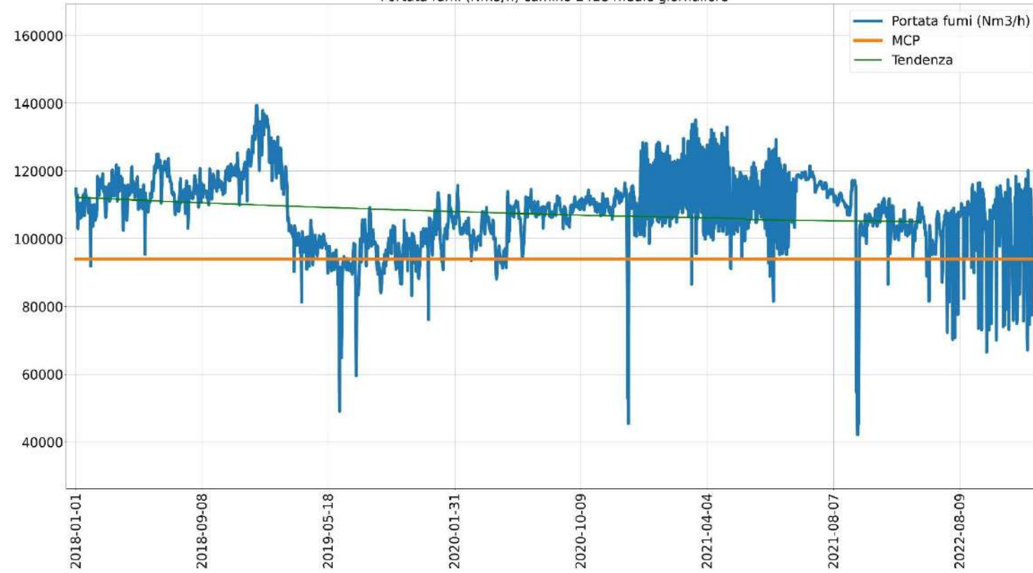
Portata fumi (Nm 3 /h) camino E428 medie giornaliere
