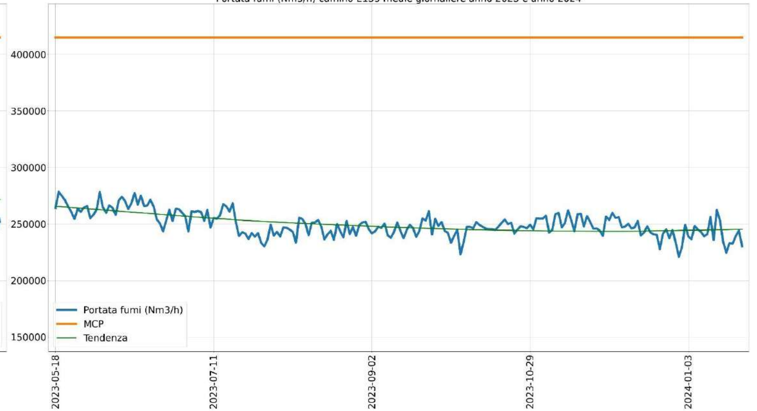
Portata fumi (Nm 3 /h) camino E135 medie giornaliere anno 2023 e anno 2024
