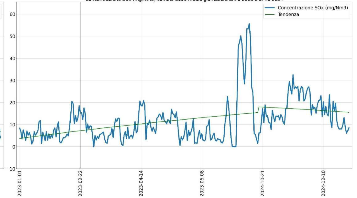
Concentrazione SO x (mg/Nm 3 ) camino E111 medie giornaliere anno 2023 e anno 2024
