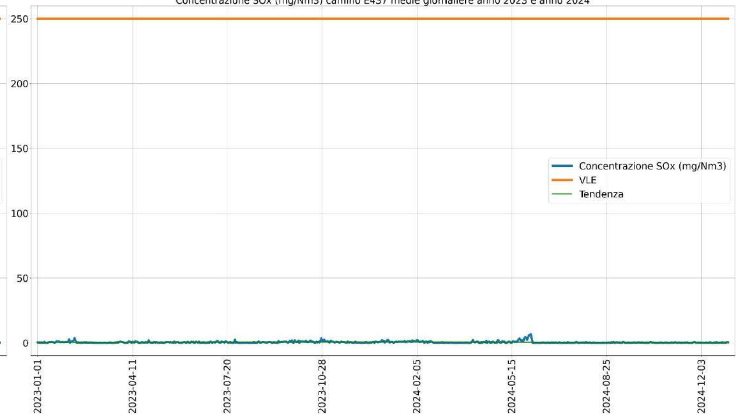
Concentrazione SOx (mg/Nm3) camino E437 medie giornaliere anno 2023 e anno 2024
