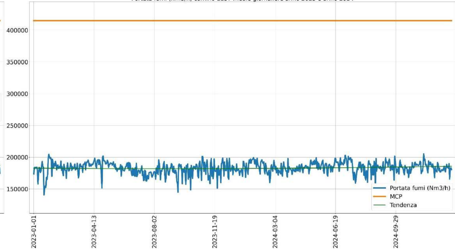
Portata fumi (Nm 3 /h) camino E137 medie giornaliere anno 2023 e anno 2024
