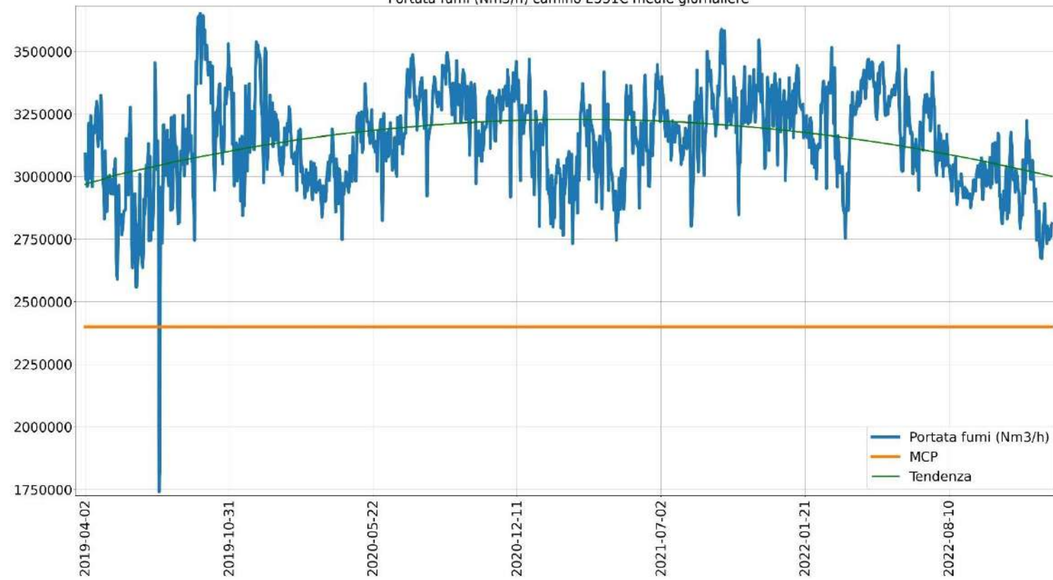
Portata fumi (Nm3/h) camino E551C medie giornaliere
