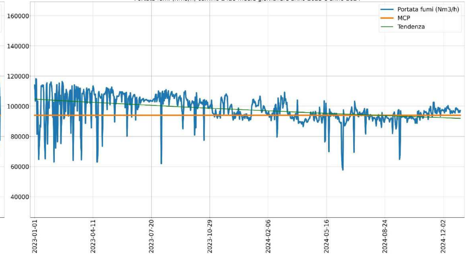
Portata fumi (Nm 3 /h) camino E428 medie giornaliere anno 2023 e anno 2024
