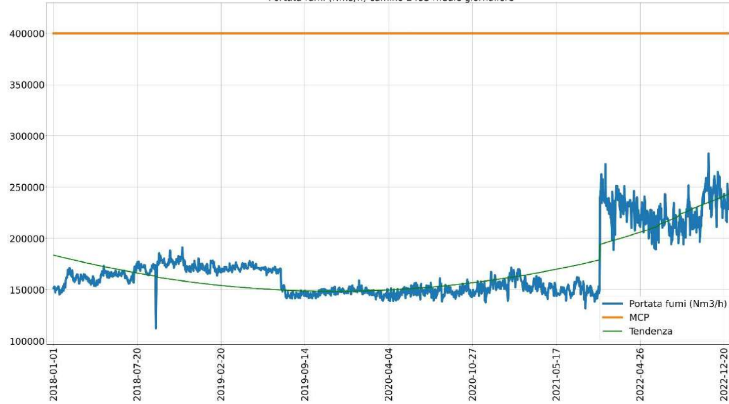
Portata fumi (Nm 3 /h) camino E435 medie giornaliere
