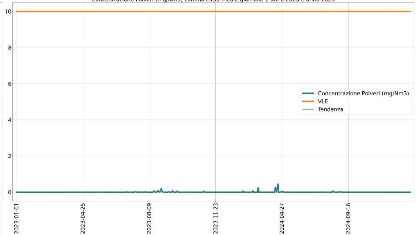
Concentrazione Polveri (mg/Nm 3 ) camino E435 medie giornaliere anno 2023 e anno 2024
