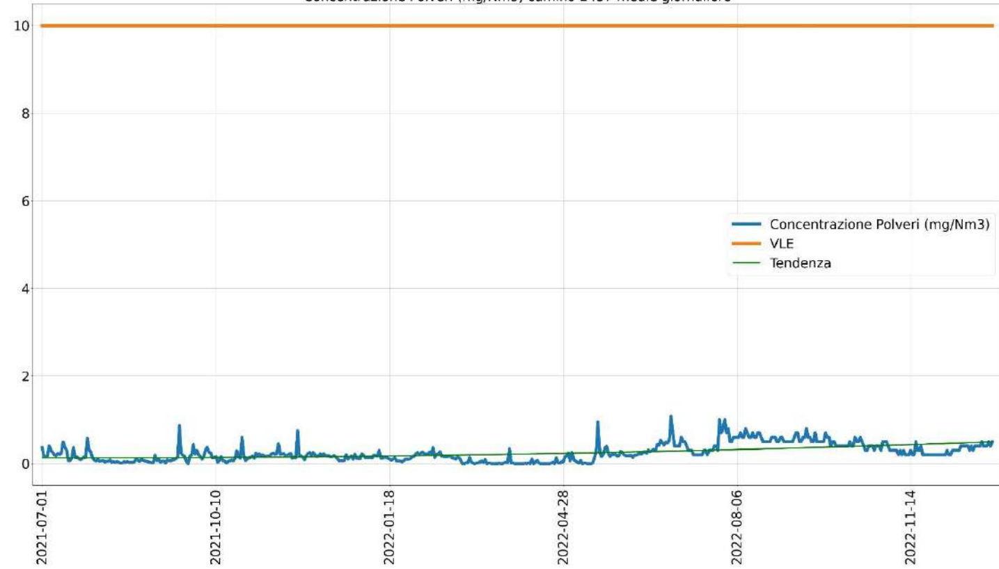
Concentrazione Polveri (mg/Nm 3 ) camino E437 medie giornaliere
