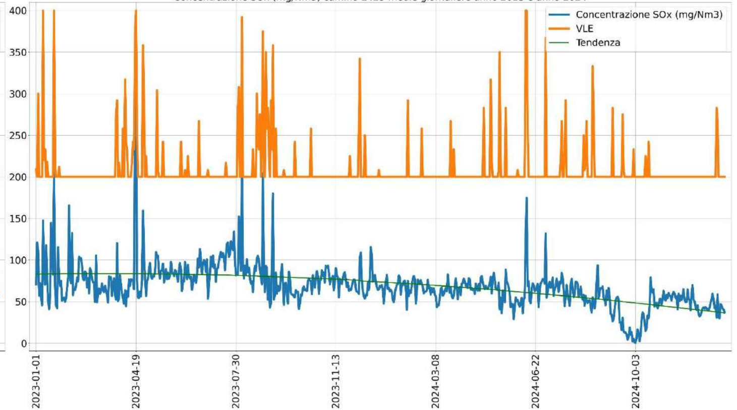
Concentrazione SOx (mg/Nm3) cammino E425 medie giornaliere anno 2023 e anno 2024
