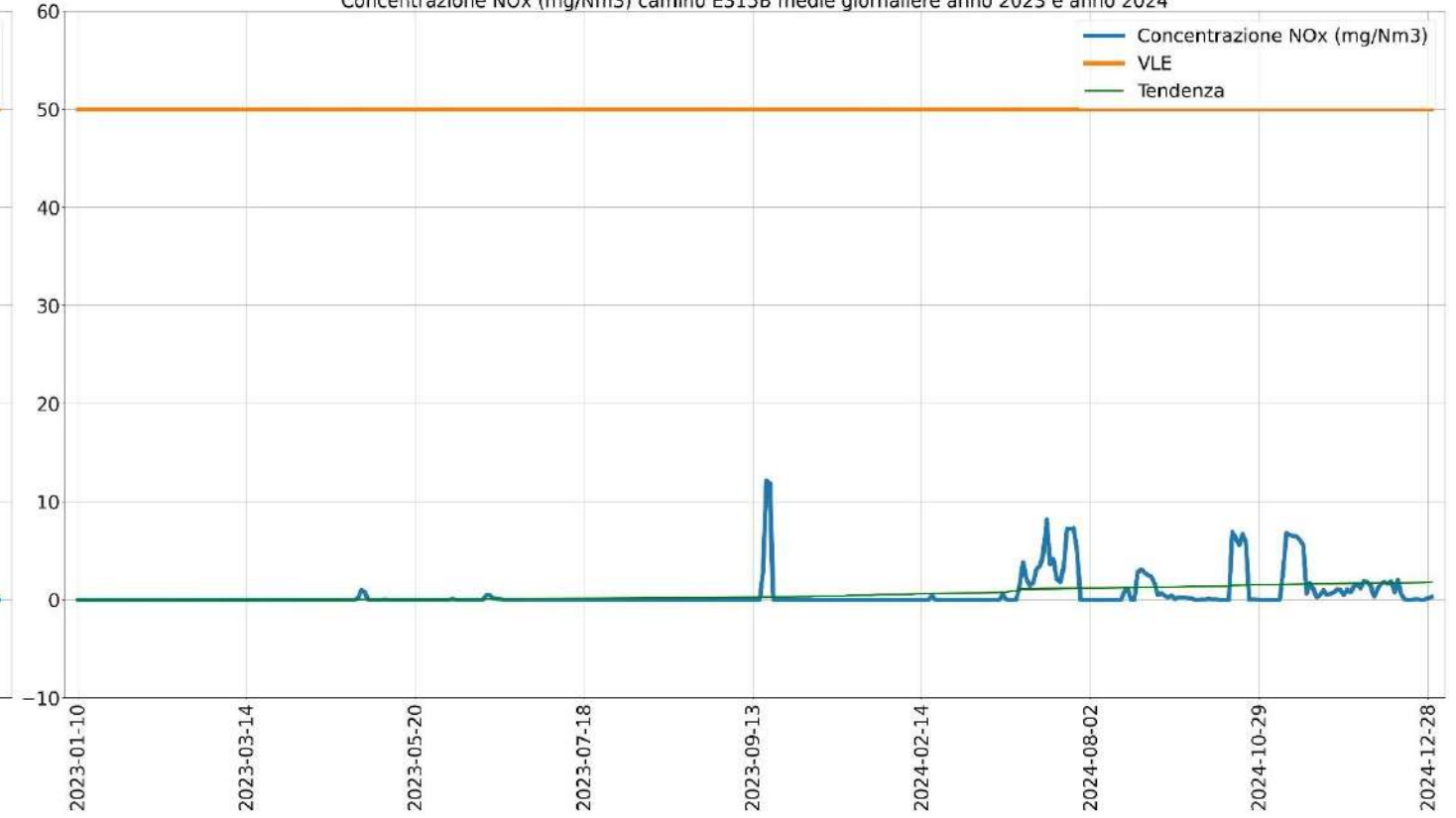
Concentrazione NOx (mg/Nm3) camino E315B medie giornaliere anno 2023 e anno 2024
