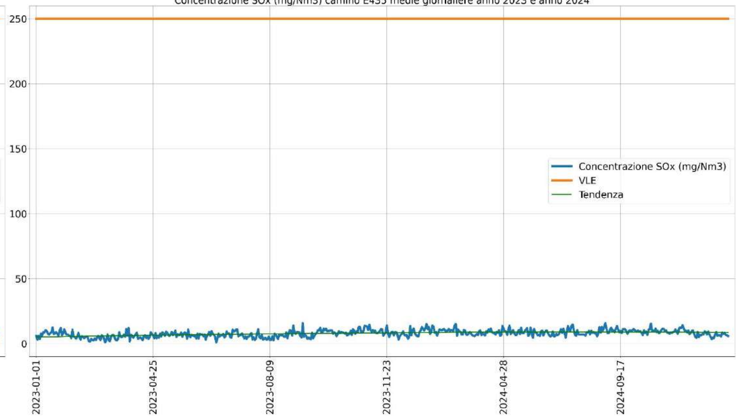
Concentrazione SOx (mg/Nm3) cammino E435 medie giornaliere anno 2023 e anno 2024
