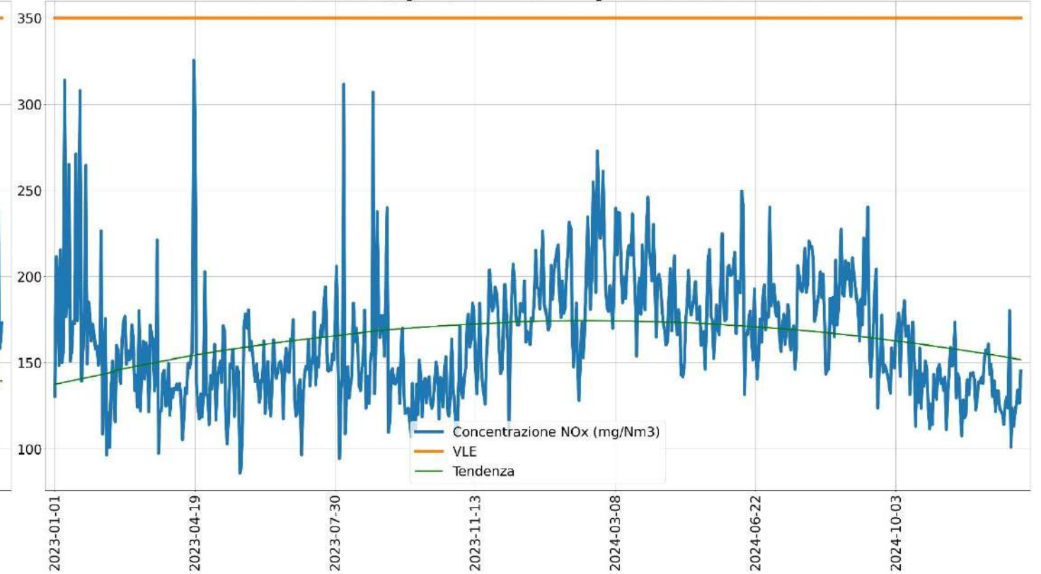
Concentrazione NOx (mg/Nm3) cammino E425 medie giornaliere anno 2023 e anno 2024
