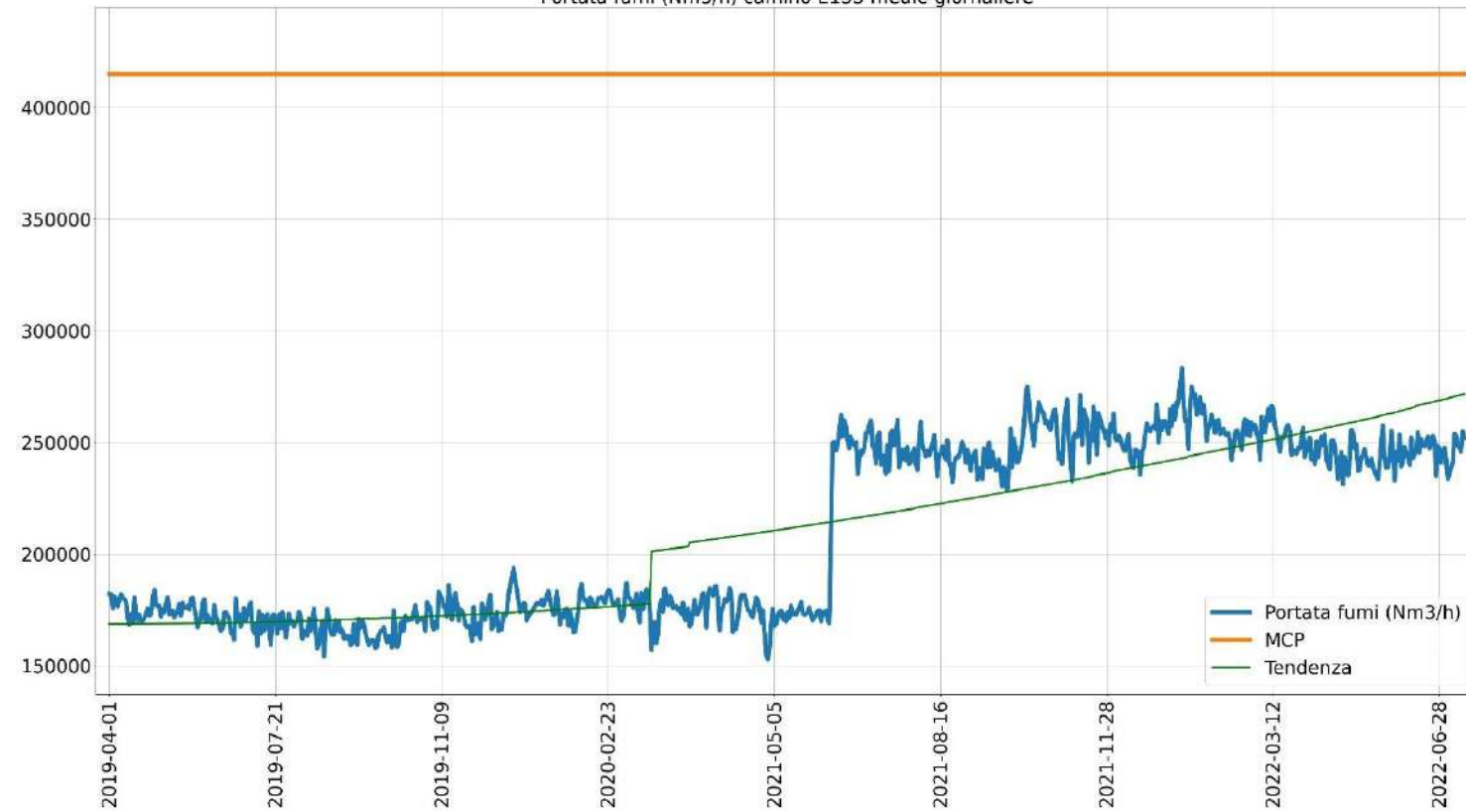
Portata fumi (Nm 3 /h) camino E135 medie giornaliere
