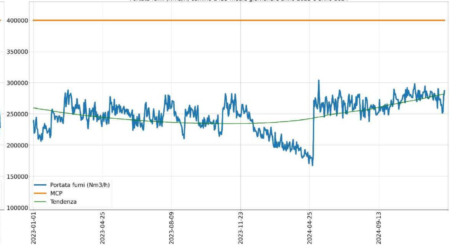
Portata fumi (Nm 3 /h) camino E435 medie giornaliere anno 2023 e anno 2024
