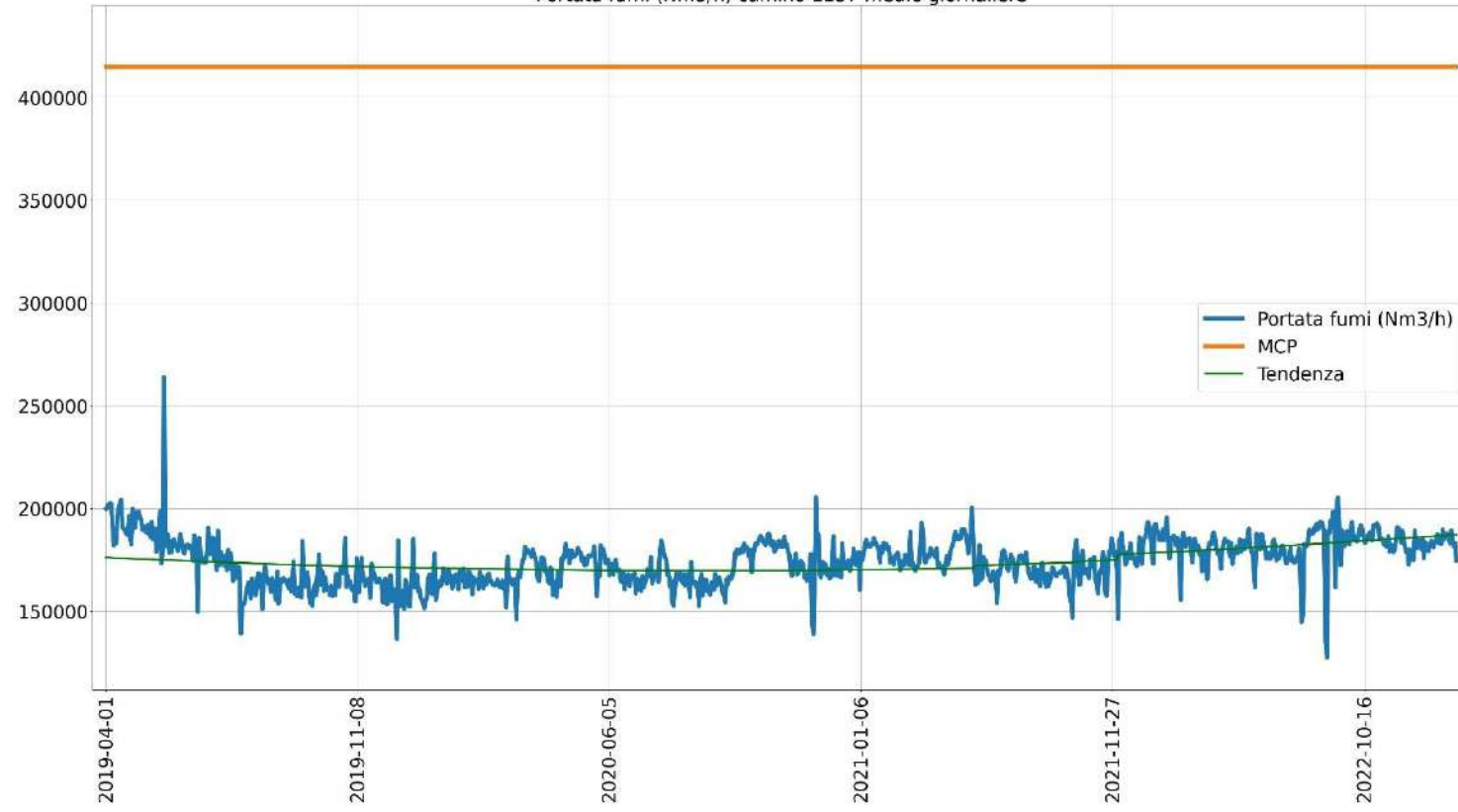
Portata fumi (Nm 3 /h) camino E137 medie giornaliere
