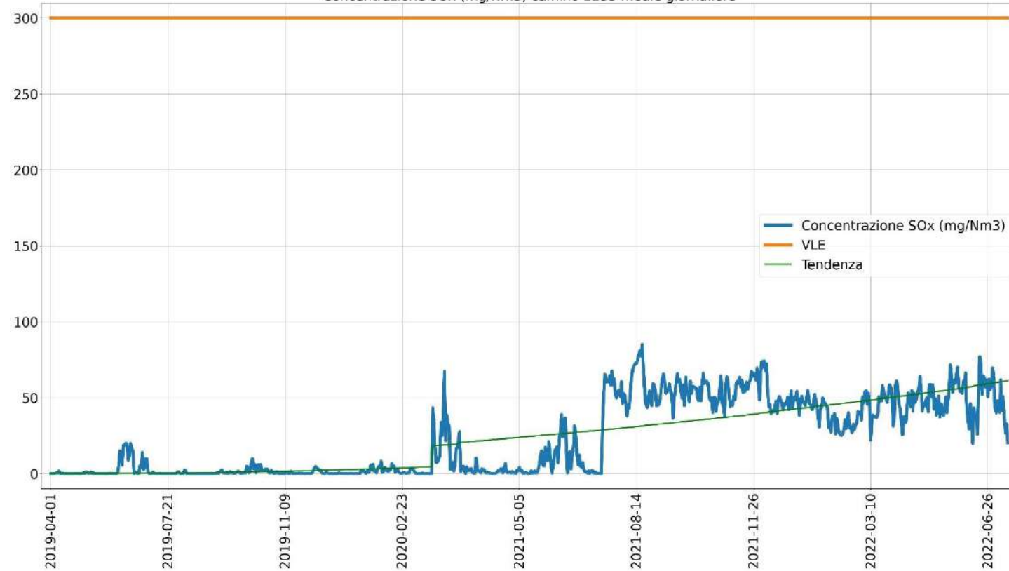
Concentrazione SOx (mg/Nm3) cammino E135 medie giornaliere
