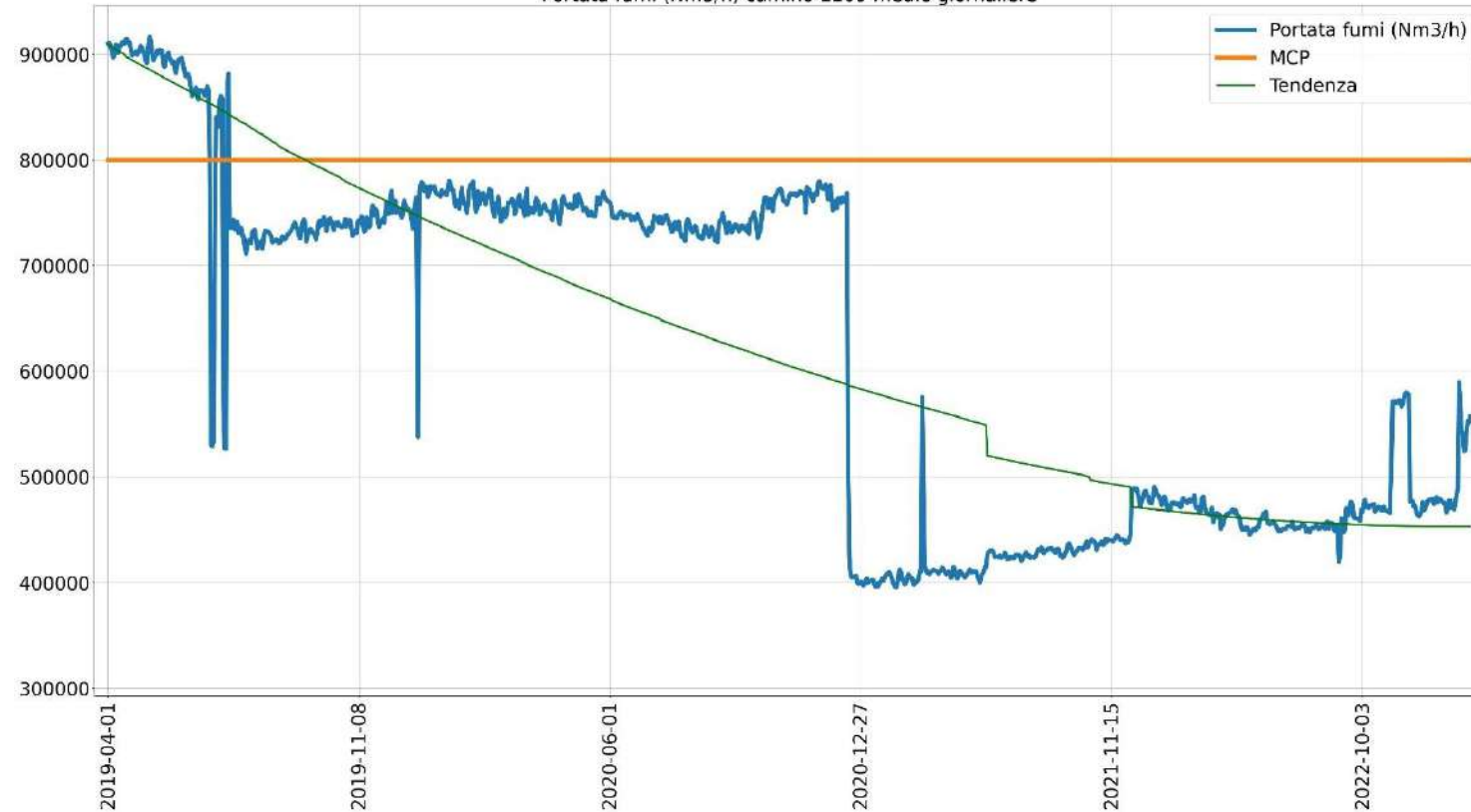
Portata fumi (Nm3/h) camino E109 medie giornaliere
