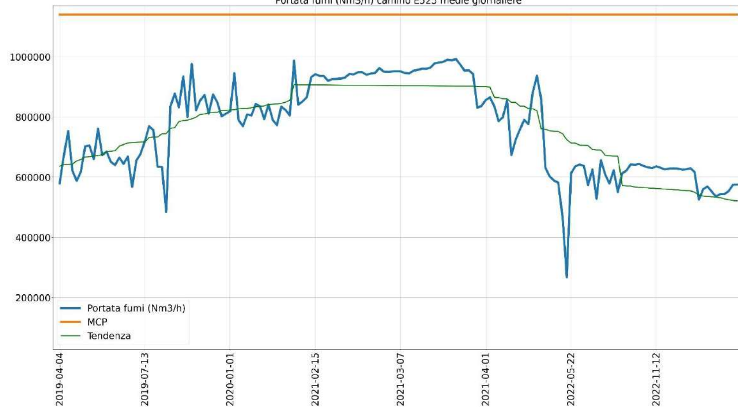
Portata fumi (Nm3/h) camino E525 medie giornaliere
