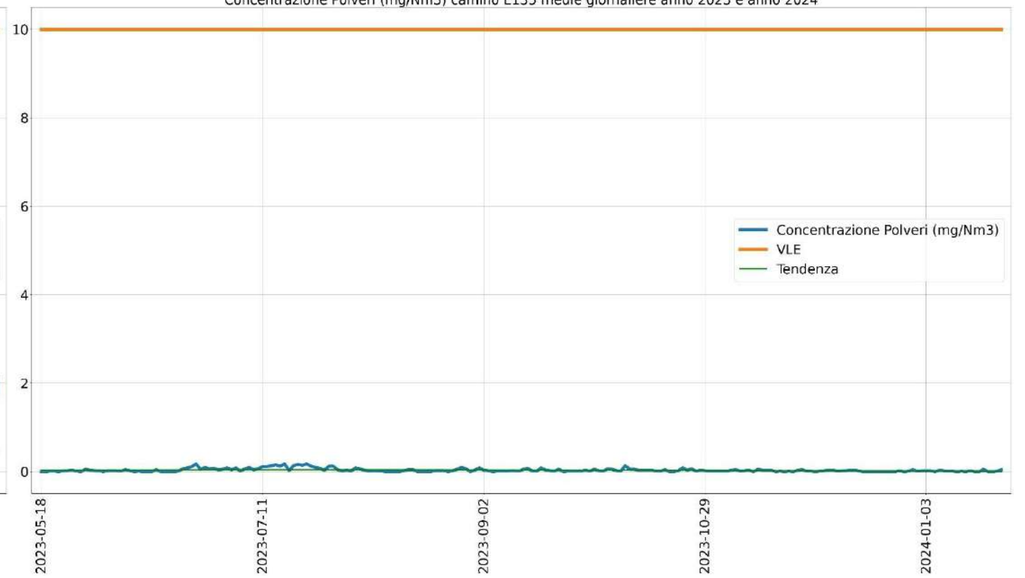
Concentrazione Polveri (mg/Nm 3 ) camino E135 medie giornaliere anno 2023 e anno 2024
