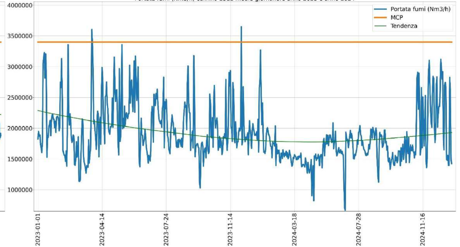
Portata fumi (Nm3/h) camino E312 medie giornaliere anno 2023 e anno 2024
