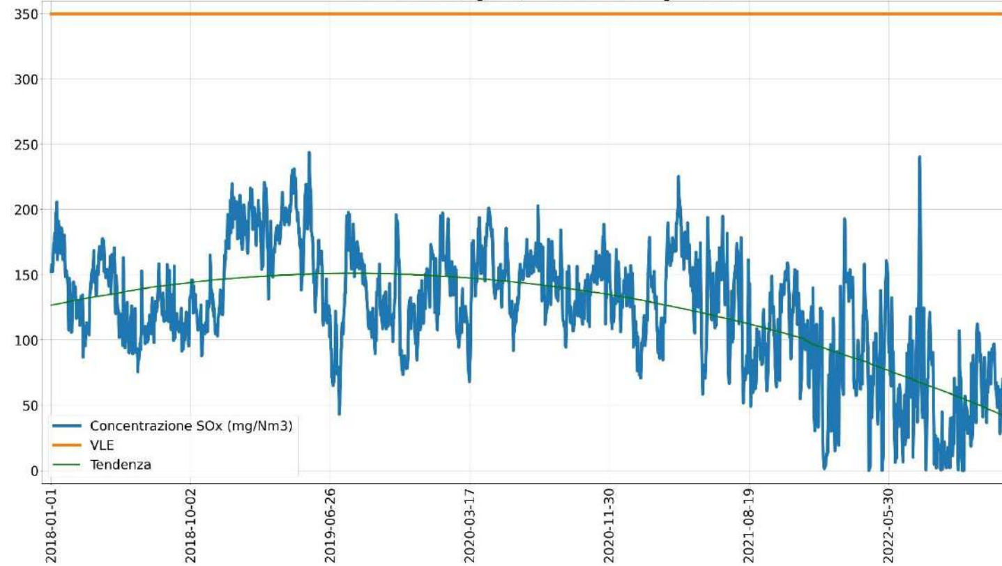
Concentrazione SOx (mg/Nm3) camino E312 medie giornaliere
