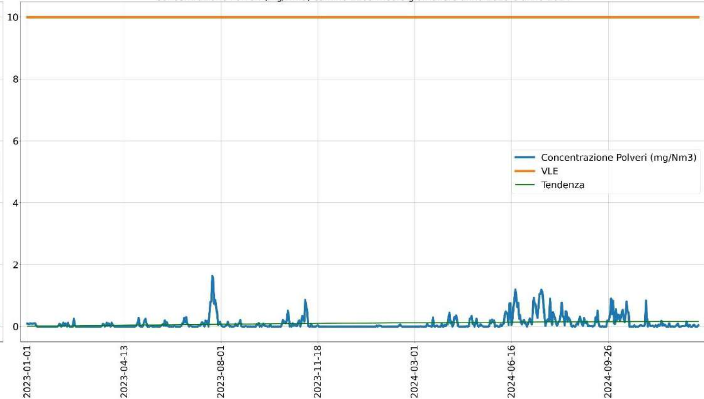
Concentrazione Polveri (mg/Nm3) camino E109 medie giornaliere anno 2023 e anno 2024
