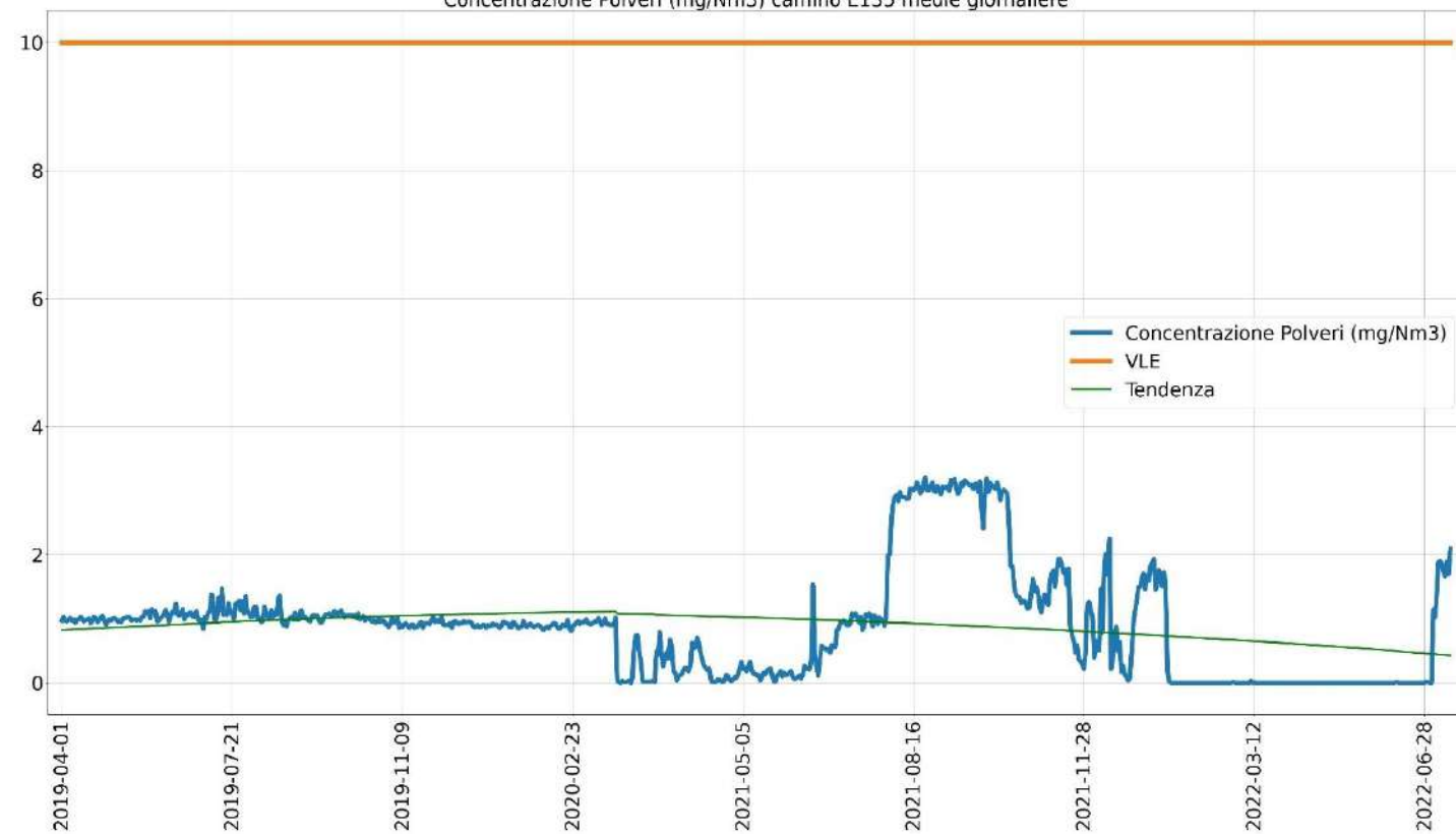
Concentrazione Polveri (mg/Nm 3 ) camino E135 medie giornaliere
