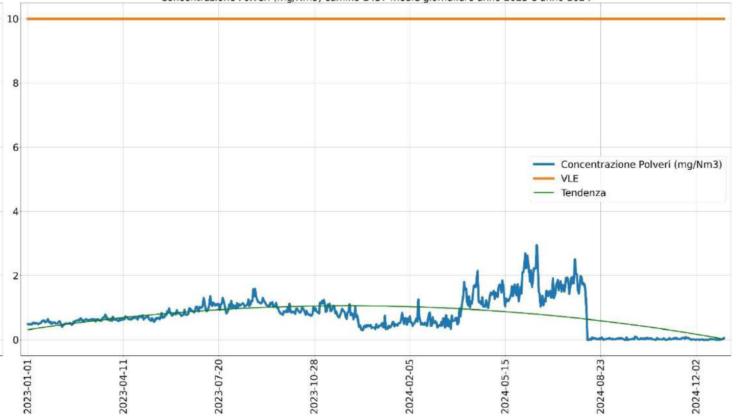
Concentrazione Polveri (mg/Nm 3 ) camino E437 medie giornaliere anno 2023 e anno 2024
