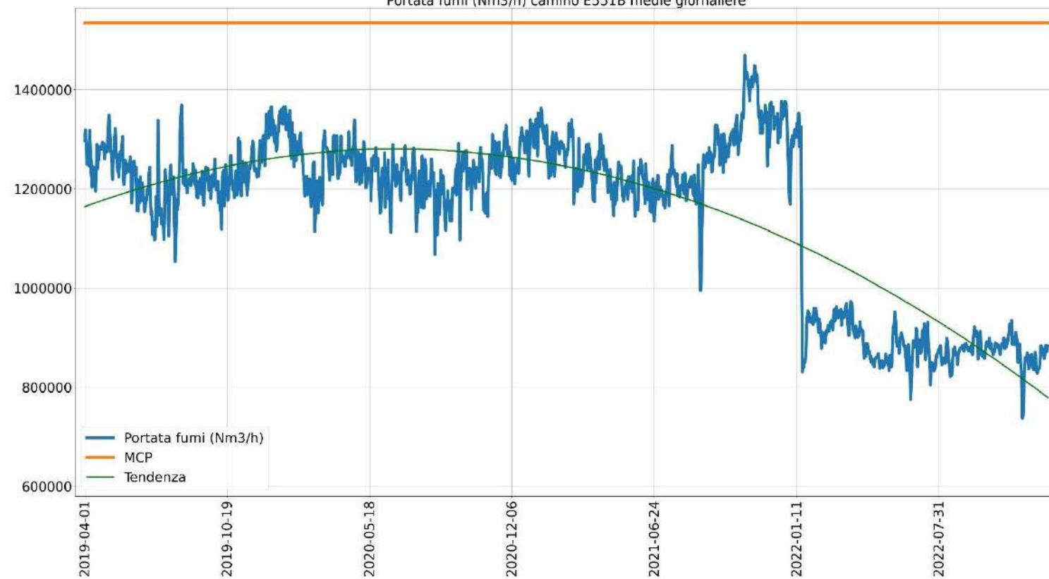
Portata fumi (Nm3/h) camino E551B medie giornaliere
