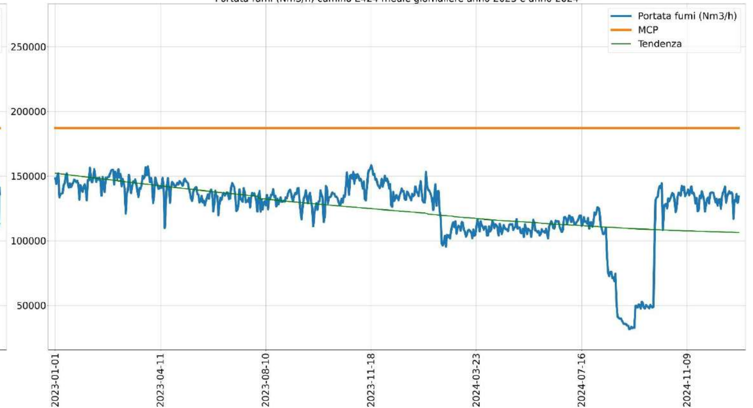
Portata fumi (Nm 3 /h) camino E424 medie giornaliere anno 2023 e anno 2024
