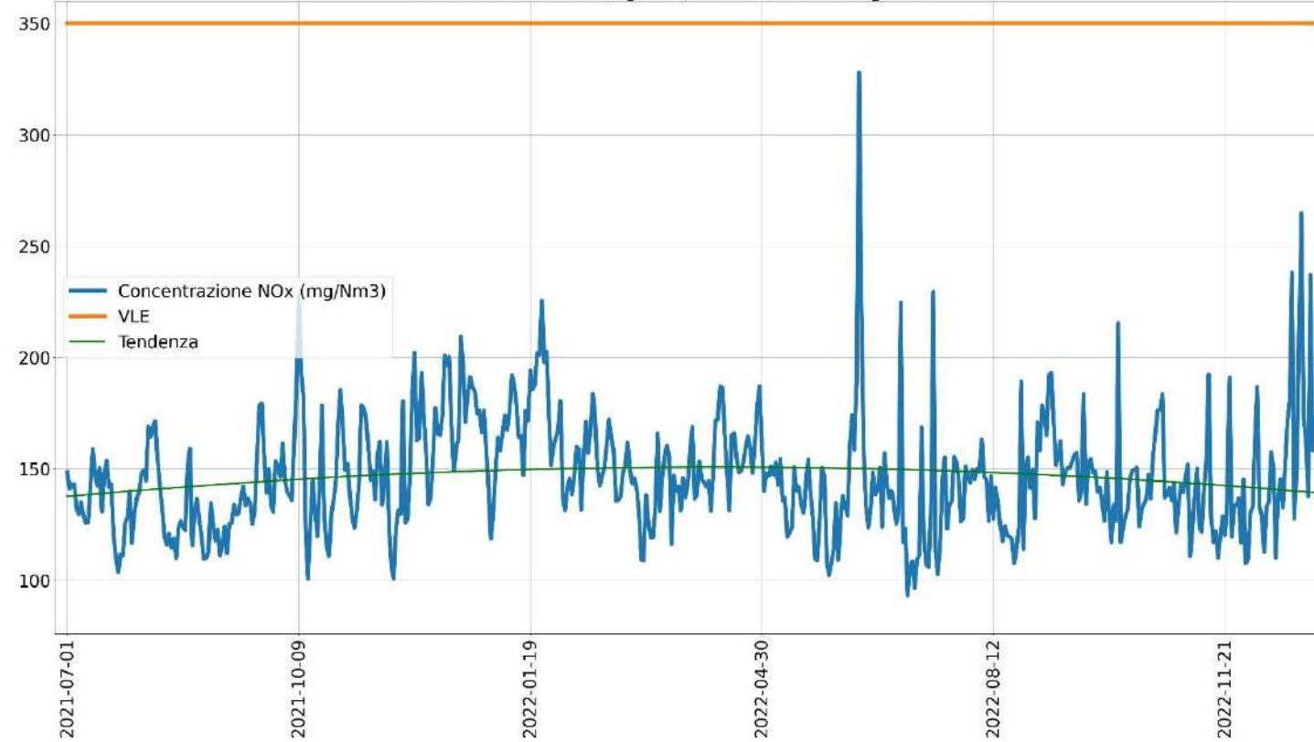
Concentrazione NOx (mg/Nm3) cammino E425 medie giornaliere
