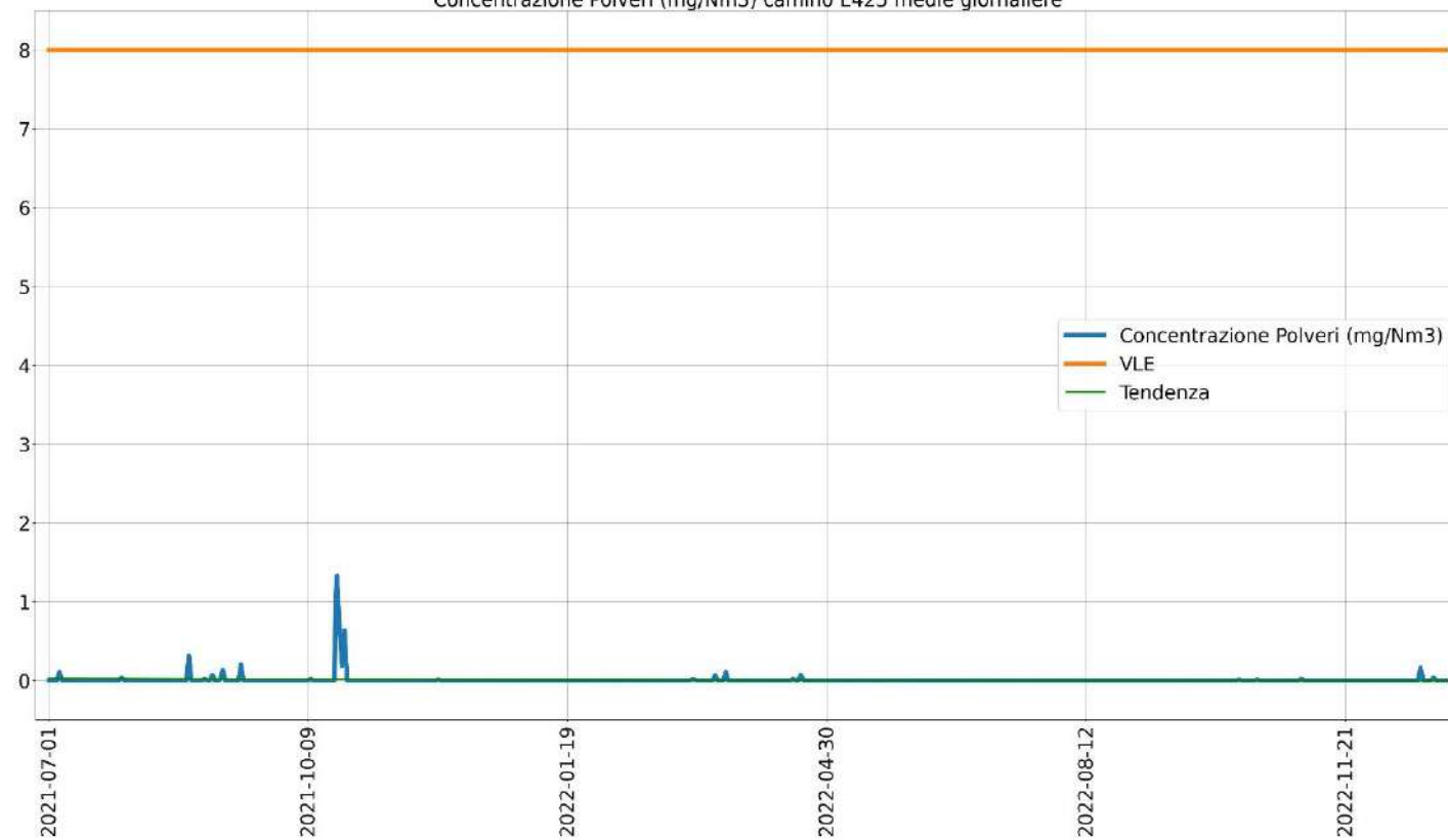
Concentrazione Polveri (mg/Nm 3 ) camino E425 medie giornaliere
