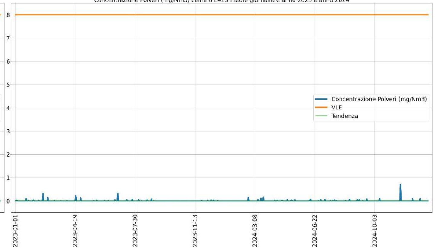
Concentrazione Polveri (mg/Nm 3 ) camino E425 medie giornaliere anno 2023 e anno 2024
