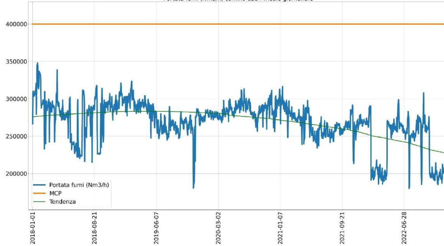
Portata fumi (Nm 3 /h) camino E324 medie giornaliere
