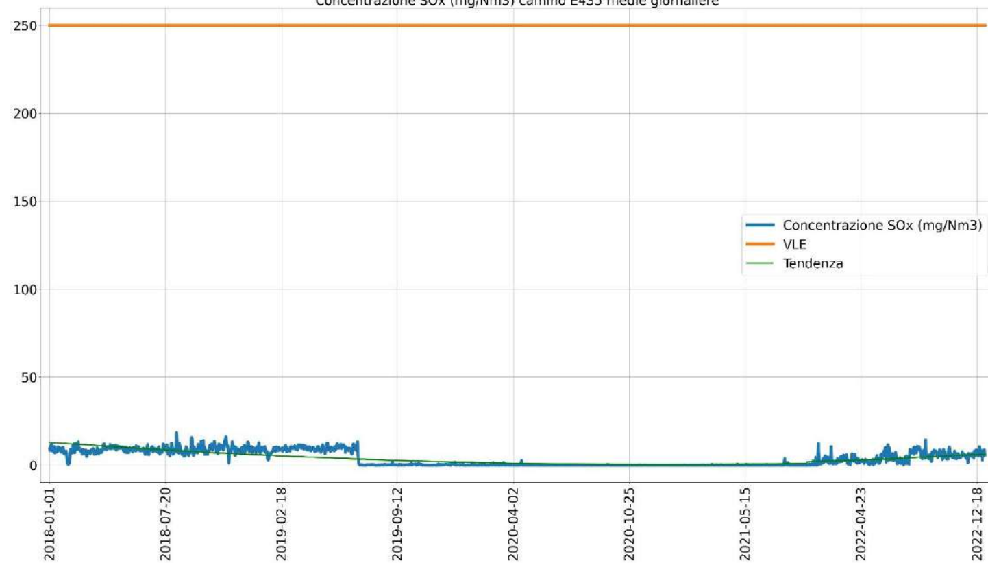
Concentrazione SOx (mg/Nm3) cammino E435 medie giornaliere
