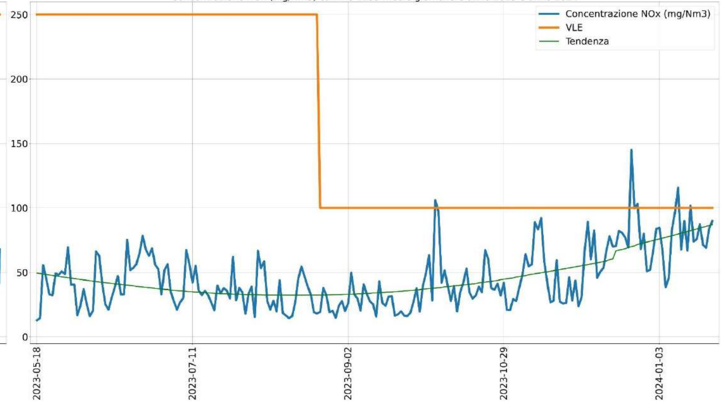
Concentrazione NOx (mg/Nm3) cammino E135 medie giornaliere anno 2023 e anno 2024
