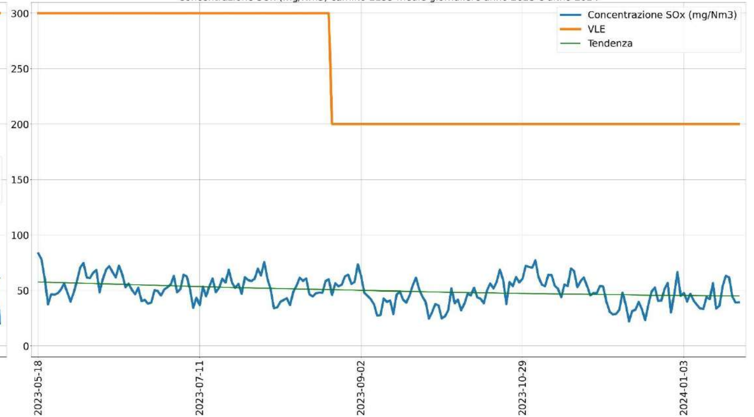
Concentrazione SOx (mg/Nm3) cammino E135 medie giornaliere anno 2023 e anno 2024
