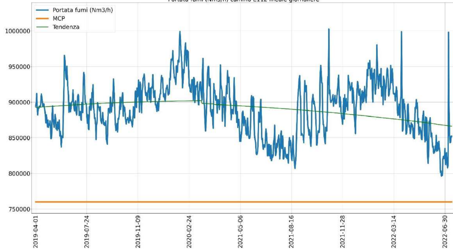
Portata fumi (Nm3/h) camino E112 medie giornaliere
