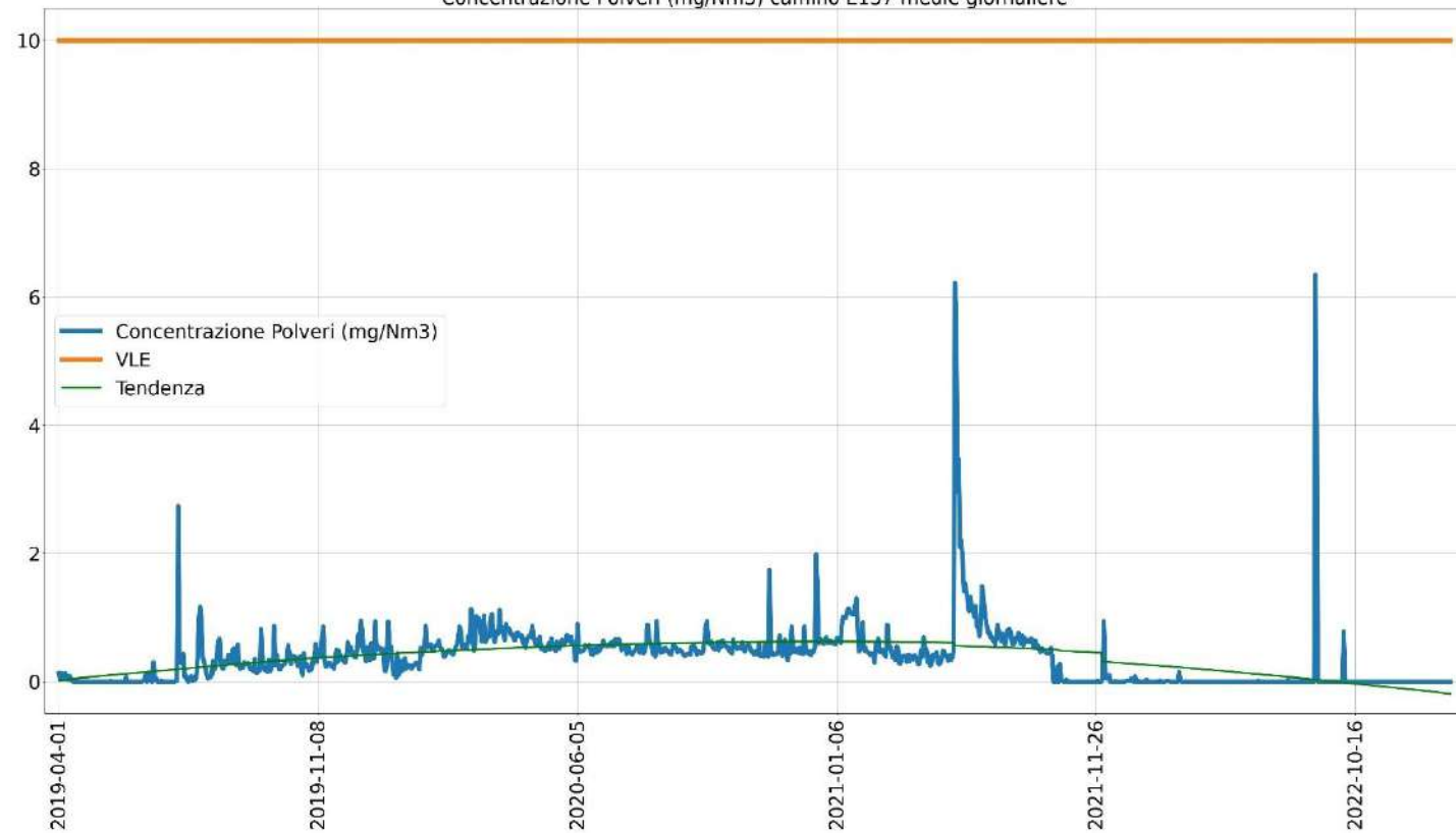
Concentrazione Polveri (mg/Nm 3 ) camino E137 medie giornaliere
